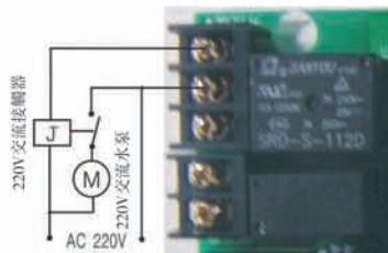
图3-8进口接增压泵的接线图
