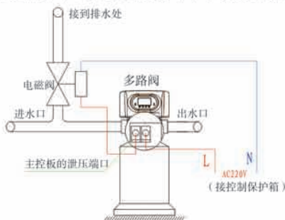
图3-10 泄压端口的接线
