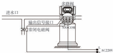
图3-3 泄压端口的接线
