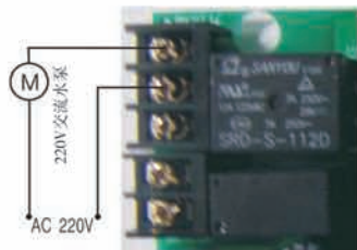
图3-7 进口接增压泵的接线图
