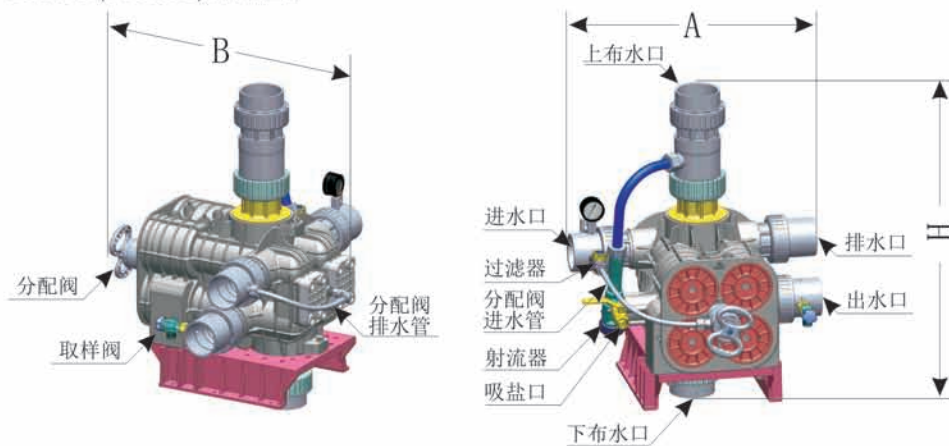
61240B(F112AS)结构图:
