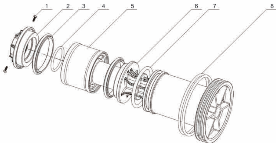
5450004 活塞零部件名称及编码:
