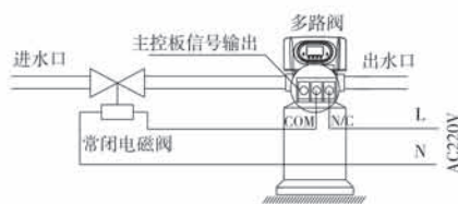
图3-2 控制进口电磁阀的接线图
