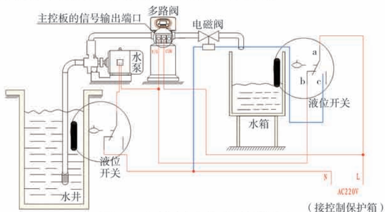
图3-5 通过水箱液位控制进水泵的接线图
