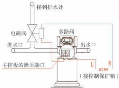
图3-10 泄压端口的接线
