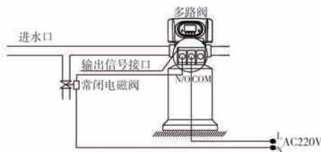
图3-3 泄压端口的接线
