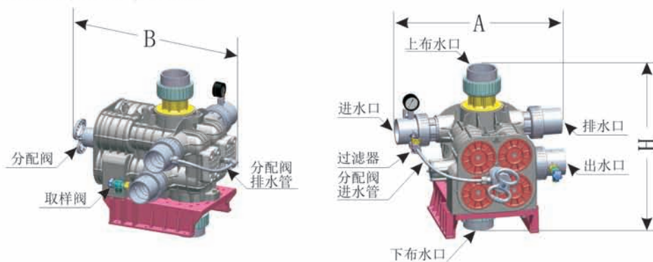
61240B(F112AS)结构图:
